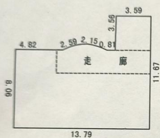
一幢一层平面图
