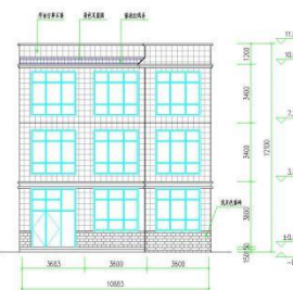
建筑西侧立面图 1:100
