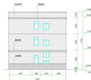
建筑南侧立面图 1:100
