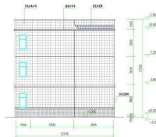
建筑北侧立面图 1:100
