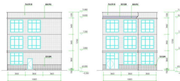
建筑东侧立面图 1:100
