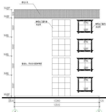
4—1 立面图 1:100
