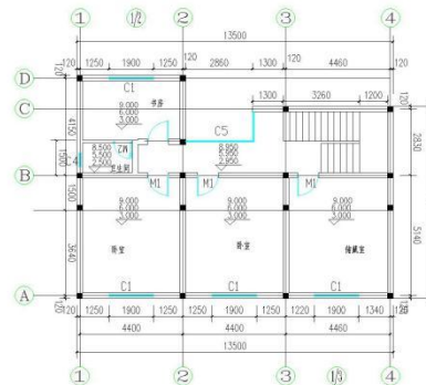
二、三、四层平面图 1:100
