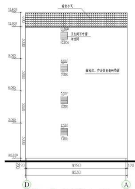
D—A 立面图 1:100
