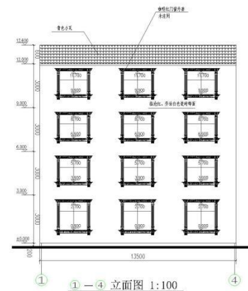
1—4 立面图 1:100
