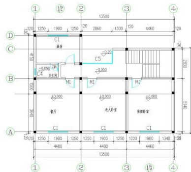
一层平面图 1:100
