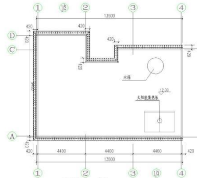
五层平面图 1:100
