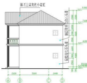
右侧立面图 1:100
