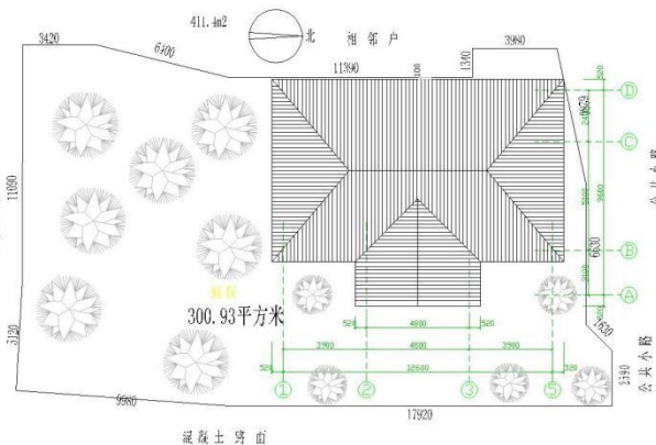
屋顶投影总平面图
