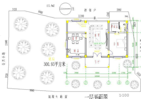
一层平面图
