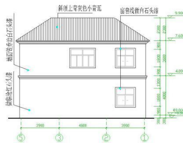
背立面图 1:100
