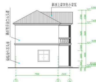
左侧立面图 1:100
