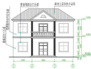
正立面图 1:100
