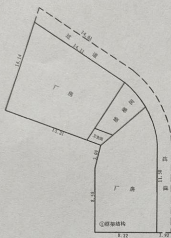
一层平面图
