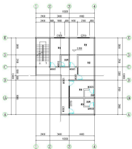
二层平面图 1:111
