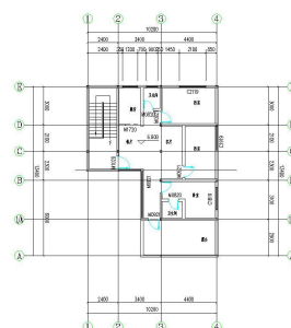
三层平面图 1:111
