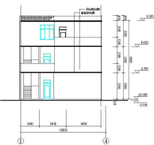
①-①剖面图 1:111
