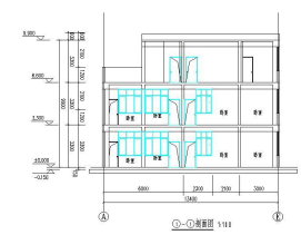
⑤-⑤剖面图 1:111
