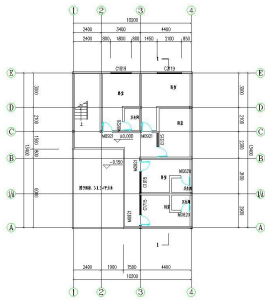
一层平面图 1:111
