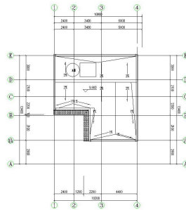
四层平面图 1:111
