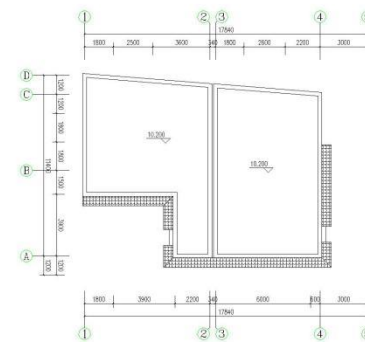
四层平面图 1:100
