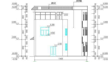
④-④剖面图 1:100
