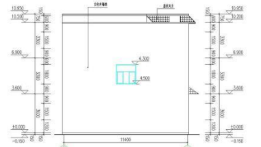
②-②剖面图 1:100
