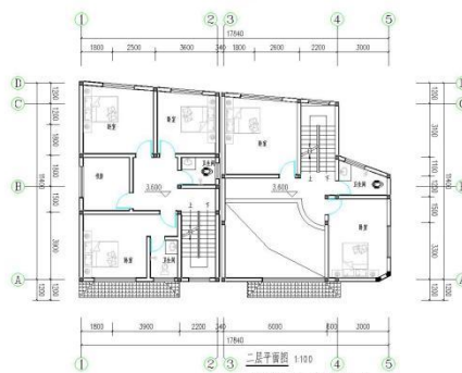
二层平面图 1:100 左P92.15m 2 , 右P68.00m 2
