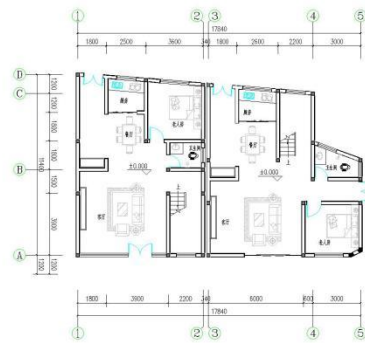
首层平面图 1:100 左P92.15m 2 , 右P93.41m 2 总建筑面积: 左P254.22m 2 , 右P226.11m 2
