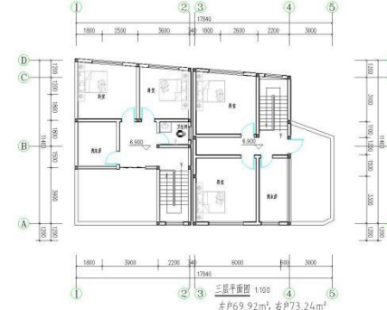
三层平面图 1:100 左P69.92m 2 , 右P73.24m 2
