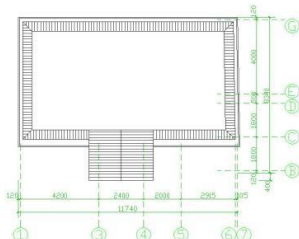
屋顶平面图 1:100
