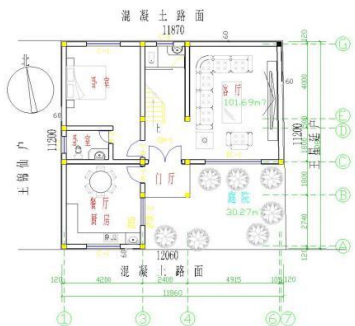
一层平面图 1:100
