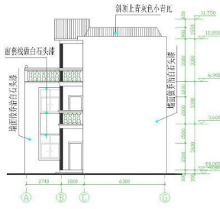
右侧立面图 1:100
