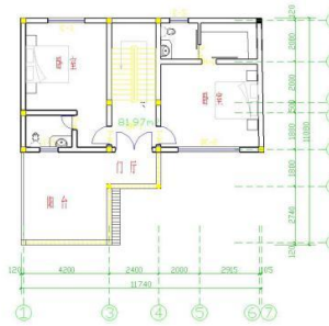
三层平面图 1:100
