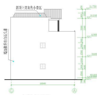
左侧立面图 1:100
