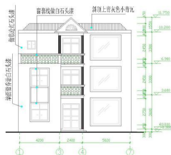
正立面图 1:100
