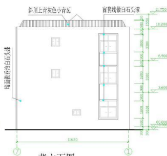
背立面图 1:100
