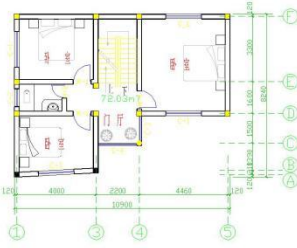
二层平面图 1:100
