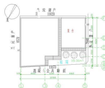
屋顶投影总平面图 1:100
