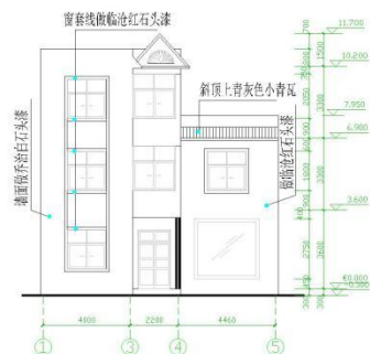
正立面图 1:100
