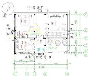
一层平面图 1:100
