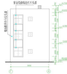
左侧立面图 1:100
