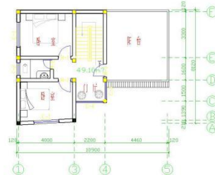
三层平面图 1:100
