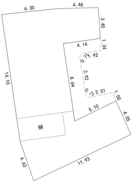
一幢二层平面图
