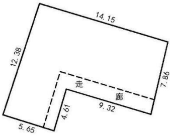
一层平面图
