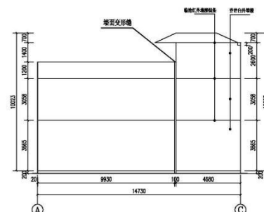
A~B立面图 1:200
