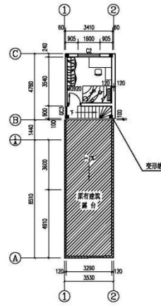
三层平面图 1:200
