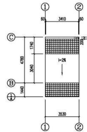
屋面平面图 1:200
