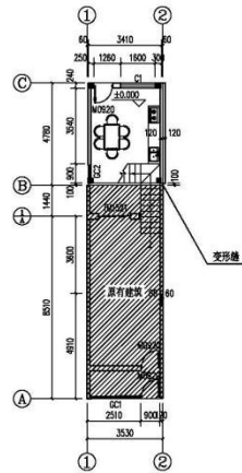
一层平面图 1:200
