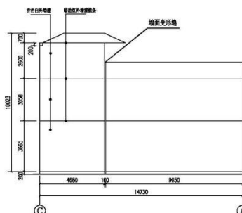
3~2立面图 1:200
