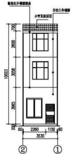
2~1立面图 1:200
