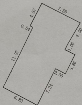
一幢一层平面图
