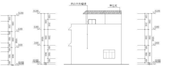
右侧立面图 1:100
