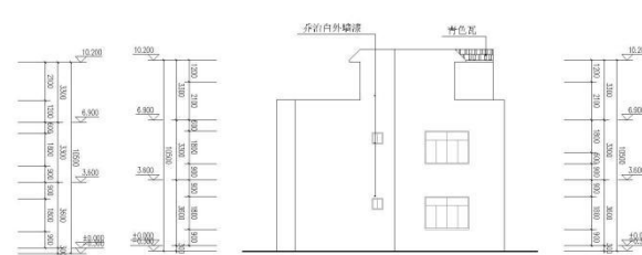
背立面图 1:100
