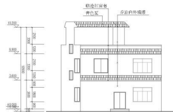
正立面图 1:100
