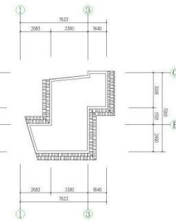
屋顶平面图 1:100
