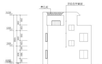
左侧立面图 1:100
