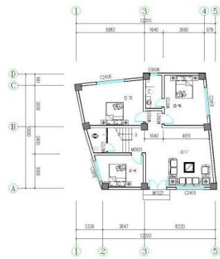
一层平面图 1:100 本层建筑面积: 108.43平方米 总建筑面积: 250.21平方米
