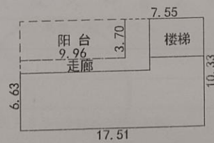
2层平面图
