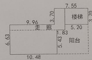
5层平面图
