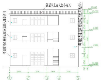
正立面图 1:100
