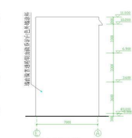
左侧立面图 1:100
