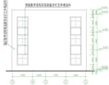
背立面图 1:100
