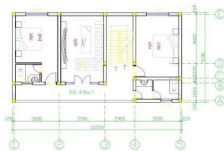
二层平面图 1:100
