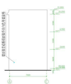
右侧立面图 1:100
