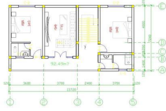
三层平面图 1:100
