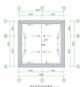
商铺四层平面布置图 1:100
