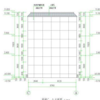
商铺C-A立面图 1:100
