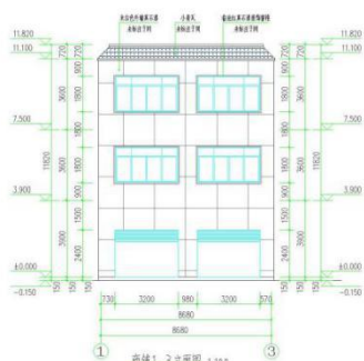
商铺1-3立面图 1:100
