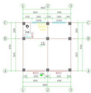
商铺一层平面布置图 1:100 本层建筑面积: 80.28平方米 总建筑面积: 240.84平方米
