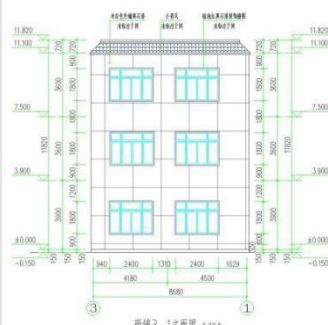
商铺3-1立面图 1:100
