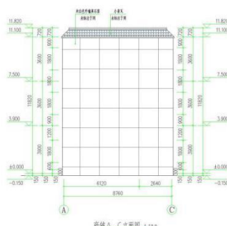
商铺A-C立面图 1:100
