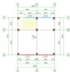
商铺二层平面布置图 1:100 本层建筑面积: 80.28平方米 总建筑面积: 240.84平方米
