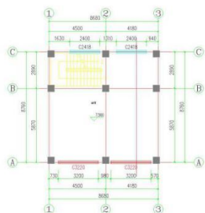
商铺三层平面布置图 1:100 本层建筑面积: 80.28平方米 总建筑面积: 240.84平方米
