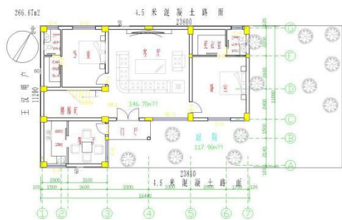
一层平面图 1:100
