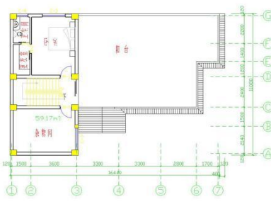
三层平面图 1:100
