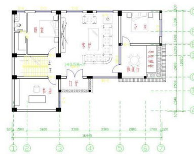
二层平面图 1:100
