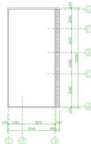
屋顶平面图 1:100
