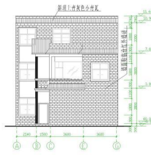
右侧立面图 1:100
