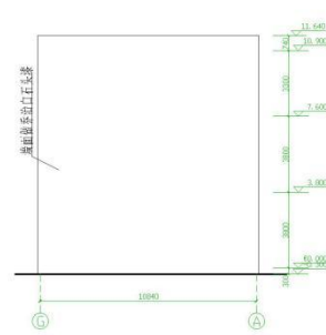
左侧立面图 1:100
