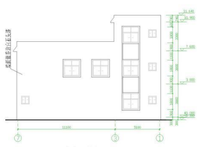
背立面图 1:100
