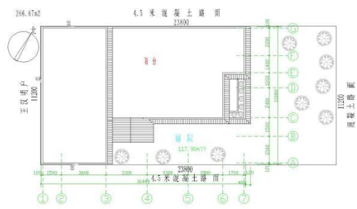
屋顶投影总平面图 1:100
