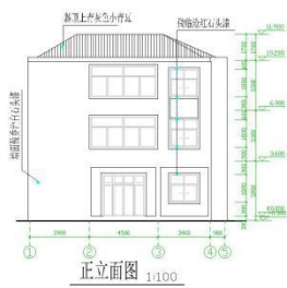
正立面图 1:100
