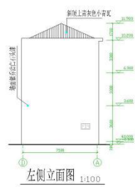
左侧立面图 1:100
