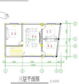
三层平面图 1:100
