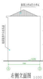
右侧立面图 1:100
