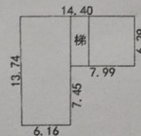
2层平面图
