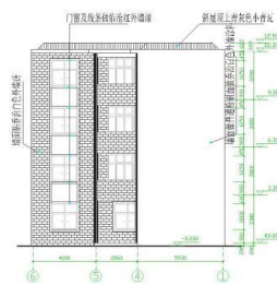
背立面图 1:100
