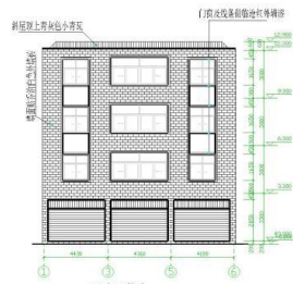
正立面图 1:100
