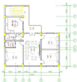
四层平面图 1:100
