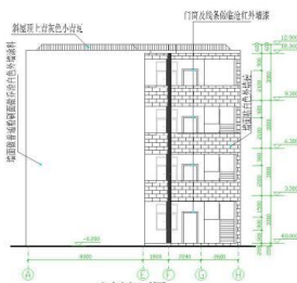
右侧立面图 1:100
