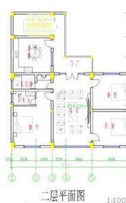
二层平面图 1:100
