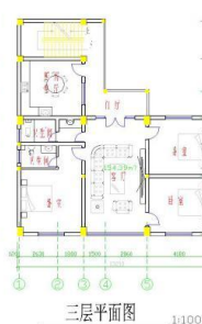
三层平面图 1:100
