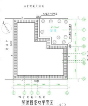
屋顶投影总平面图 1:100
