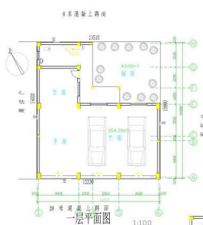
一层平面图 1:100
