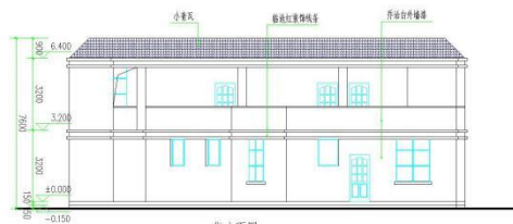
立面图 1:100
