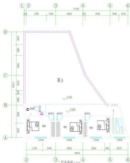
一层平面图 1:100 本层建筑基底 82.17 平方米
