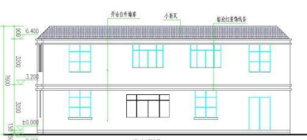
正立面图 1:100
