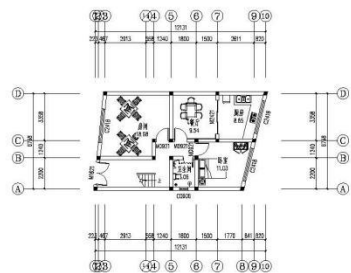
一层平面图 1:100 总建筑面积: 79.62平方米 建筑占地面积: 236.49平方米
