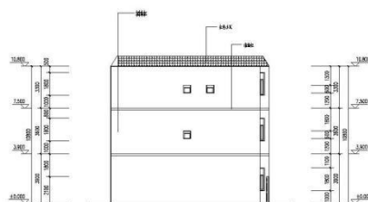
背立面 1:100
