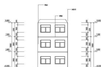
右立面 1:100
