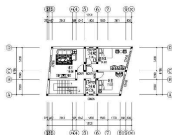
二层平面图 1:100 总建筑面积: 79.62平方米
