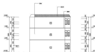
正立面 1:100
