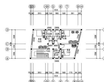
三层平面图 1:100 总建筑面积: 79.62平方米
