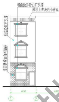
正立面图 1:100
