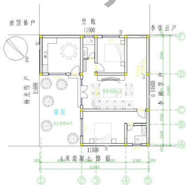
一层平面图 1:100
