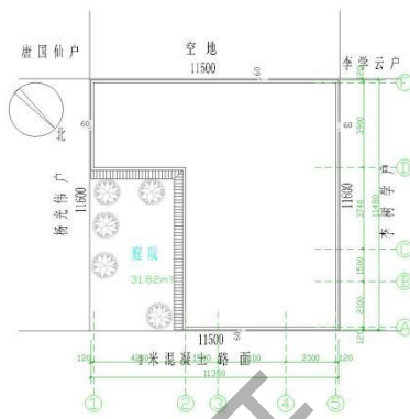
屋顶投影总平面图 1:100
