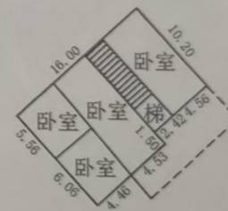
1幢3层平面图
