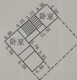
1幢2层平面图
