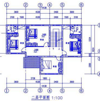
二层平面图 1:100
