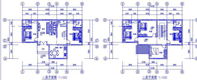
一层平面图 1:100
