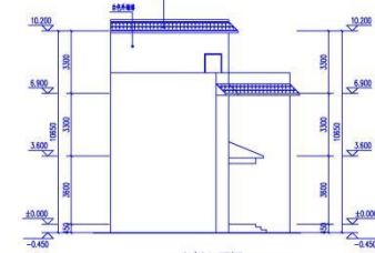
左侧立面图 1:100
