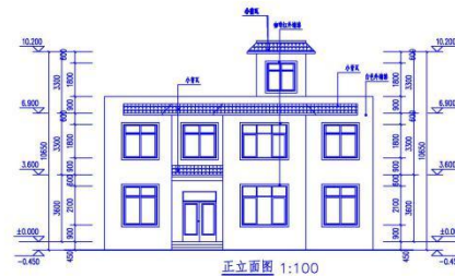
正立面图 1:100
