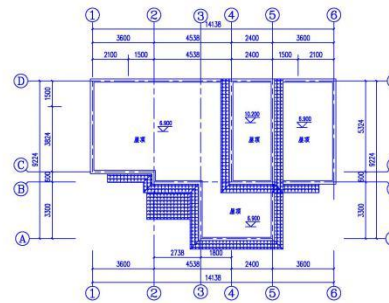
顶层平面图 1:100
