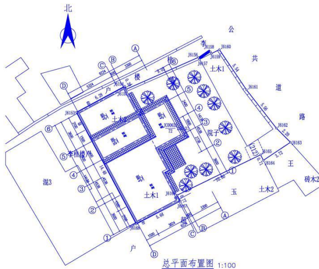
总平面布置图 1:100
