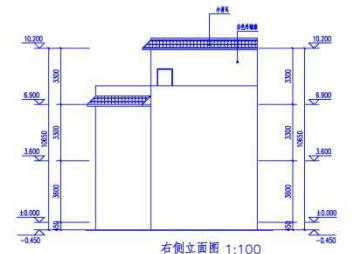
右侧立面图 1:100
