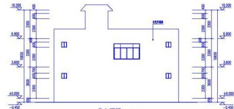
背立面图 1:100
