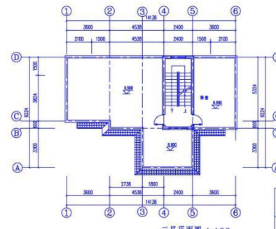
三层平面图 1:100
