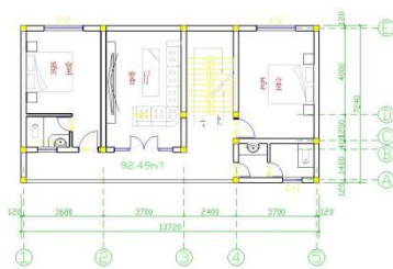
二层平面图 1:100
