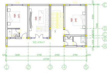
三层平面图 1:100
