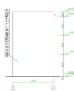
左侧立面图 1:100
