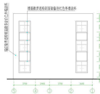
背立面图 1:100
