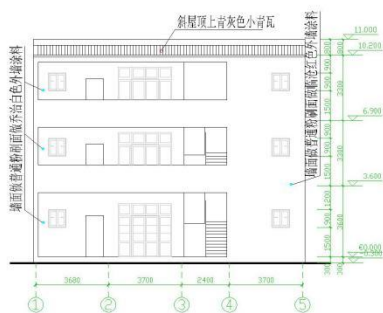
正立面图 1:100
