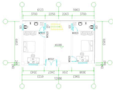
一层平面图 1:200 建筑面积: 89.11m²
