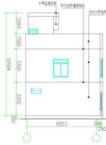
B~A立面图 1:200
