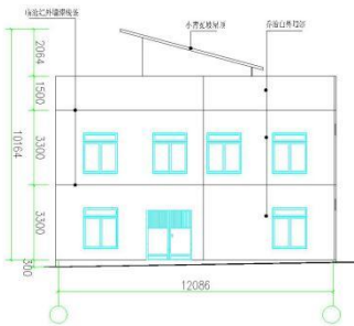
①~③立面图 1:200
