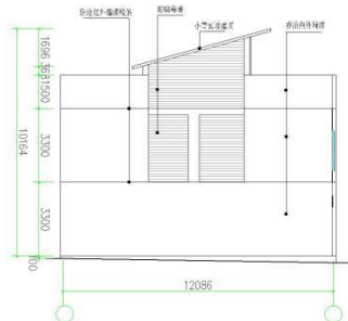
③~①立面图 1:200
