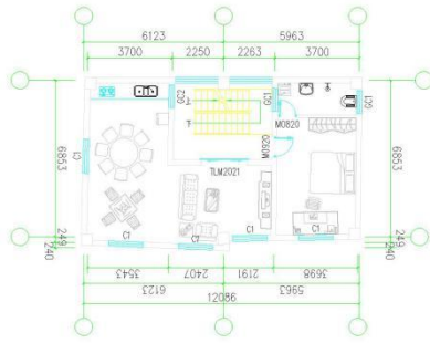
二层平面图 1:200 建筑面积: 89.11m²
