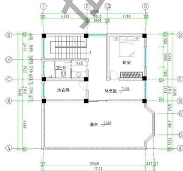
三层平面图
