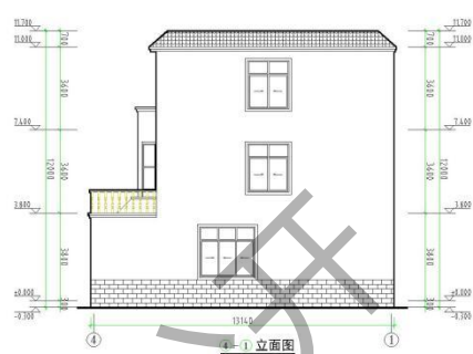
4-1 立面图
