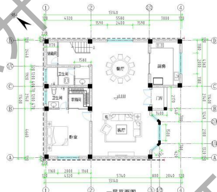
一层平面图
