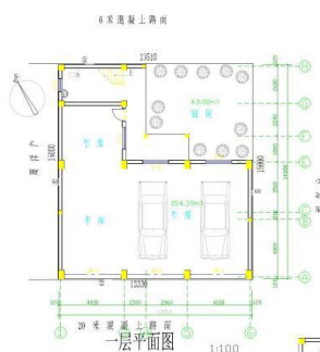
一层平面图 1:100
