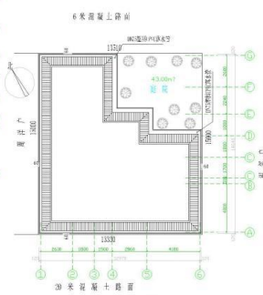
屋顶投影总平面图 1:100
