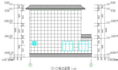
1-1剖面图 1:100
