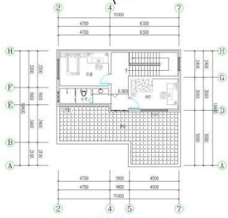
二层平面图 1:100 本层建筑面积: 61.04m²
