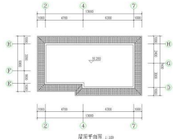
屋顶平面图 1:100
