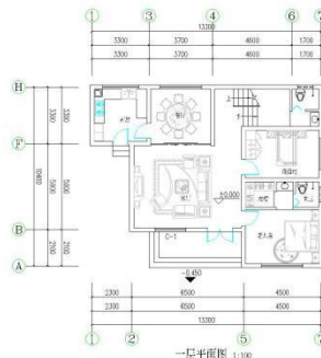
一层平面图 1:100 本层建筑面积: 114.09m² 总建筑面积: 291.97m²
