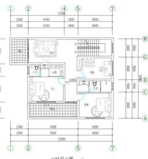
二层平面图 1:100 本层建筑面积: 116.84m²
