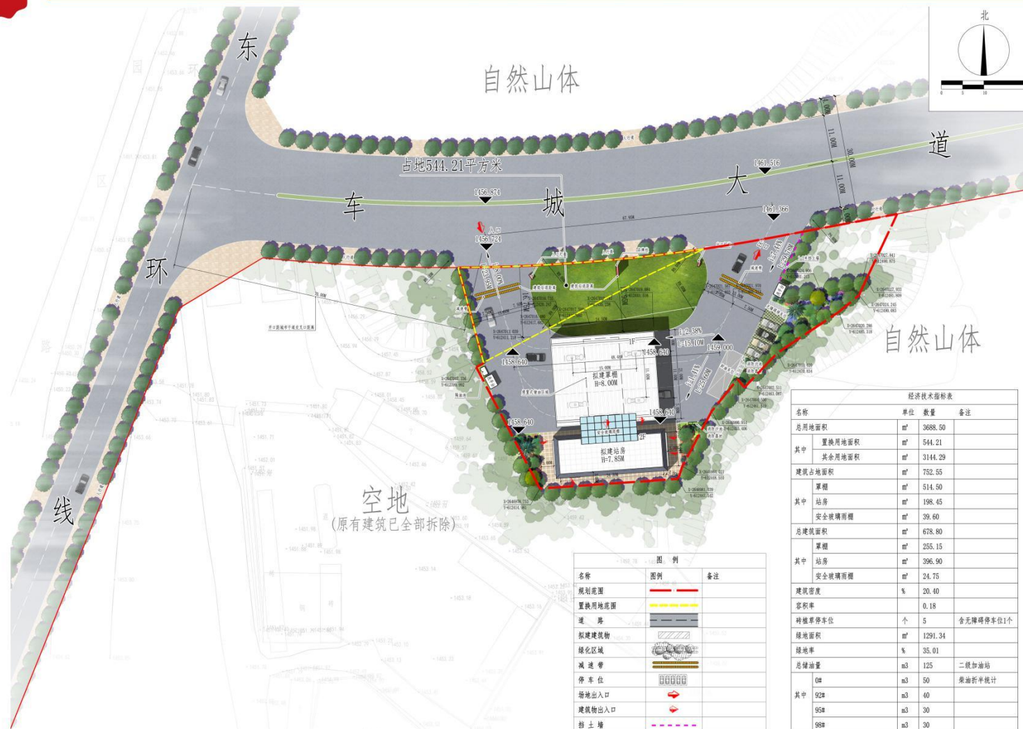
总平面图
