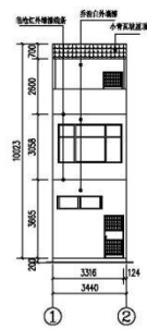
1~2立面图 1:200
