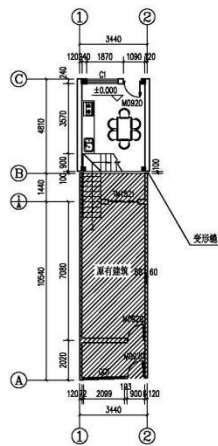
一层平面图 1:200 原有建筑面积: 46.75m 2 新建建筑面积: 16.55m 2
