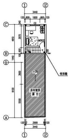
三层平面图 1:200 原有建筑面积: 0.00m 2 新建建筑面积: 16.55m 2
