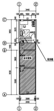
二层平面图 1:200 原有建筑面积: 24.12m 2 新建建筑面积: 16.55m 2
