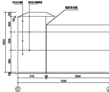
C~A立面图 1:200
