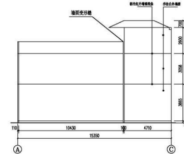
A~C立面图 1:200
