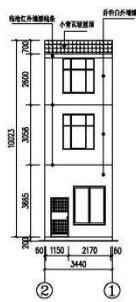
2~1立面图 1:200
