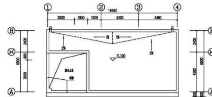
屋顶平面图 1:100
