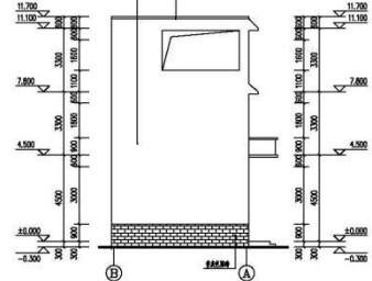
④-①轴立面图 1:100
