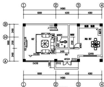
一层平面图 1:100 总建筑面积:168.00m 2 新建建筑占地面积:101.31m 2
