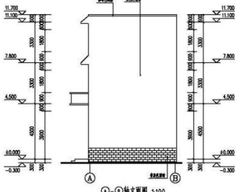
①-④轴立面图 1:100
