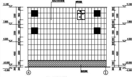
④-①轴立面图 1:100
