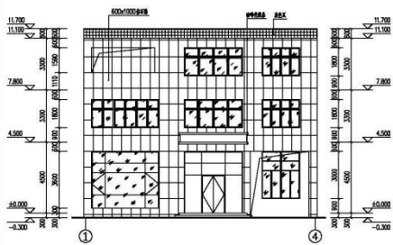
①-④轴立面图 1:100
