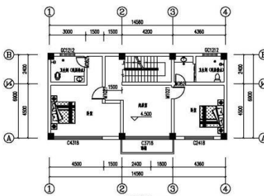
二层平面图 1:100 总建筑面积:168.00m 2 新建建筑占地面积:101.31m 2
