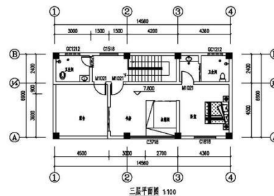
三层平面图 1:100 总建筑面积:168.00m 2 新建建筑占地面积:101.31m 2
