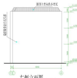
左侧立面图 1:100
