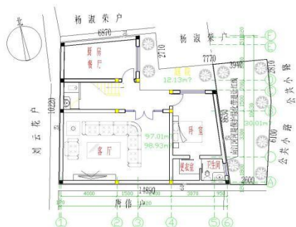
一层平面图 1:100
