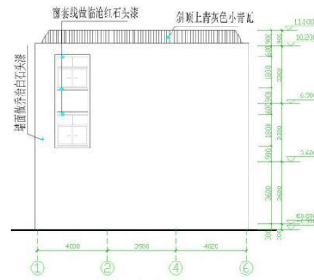
背立面图 1:100
