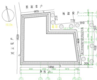
屋顶平面图 1:100
