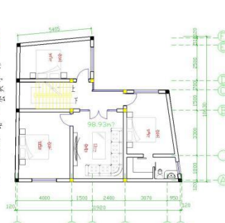
二层平面图 1:100
