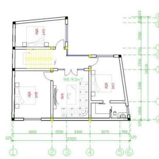
三层平面图 1:100
