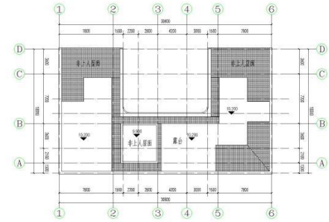
茶苑路民宅屋顶平面图 1:100
