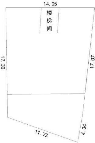
三层平面图
