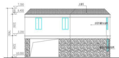
左侧立面图 1:100
