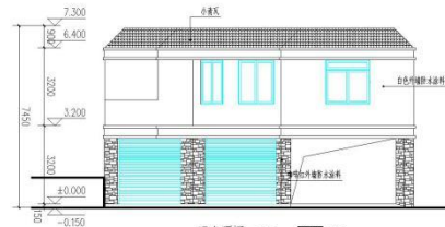
正立面图 1:100
