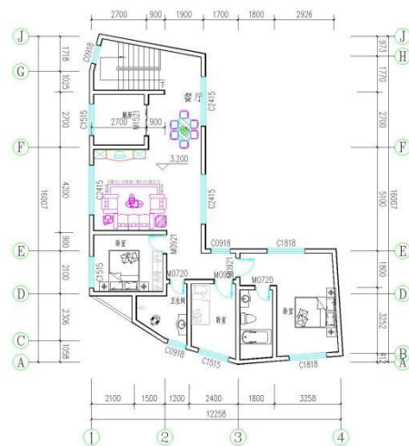
二层平面图 1:100 本层建筑面积: 115.44平方米
