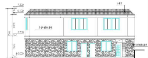
右侧立面图 1:100
