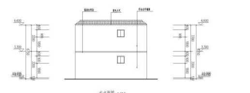
右立面图 1:100
