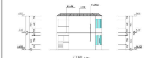
左立面图 1:100
