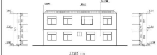
正立面图 1:100
