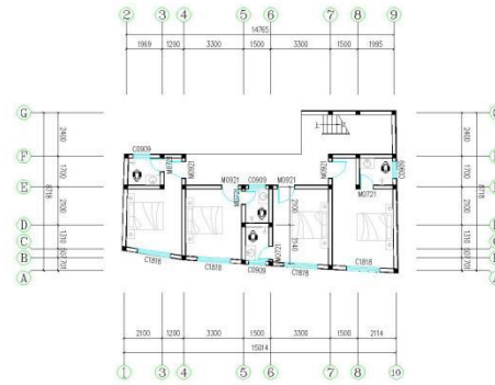
一层平面图 1:100 本层建筑面积为72.24平方米 本层占地面积为20.78平方米
