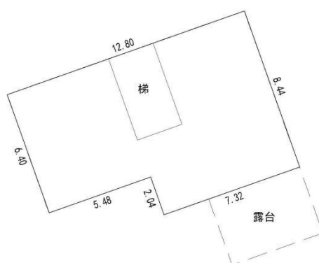
一幢二层平面图
