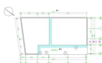
屋顶平面图 1:100
