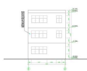
左侧立面图 1:100
