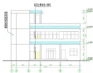
正立面图 1:100
