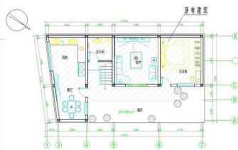
原建一层平面图 1:100
