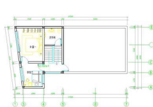
三层平面图 1:100
