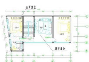
二层平面图 1:100
