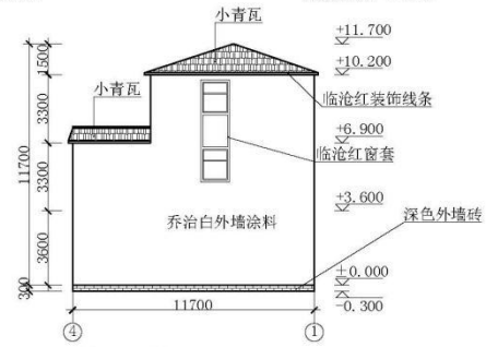
④—① 轴立面图 1:200
