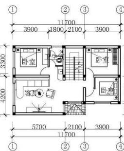
二层平面布置图 1:200
