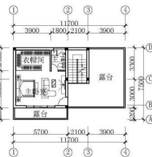
三层平面布置图 1:200
