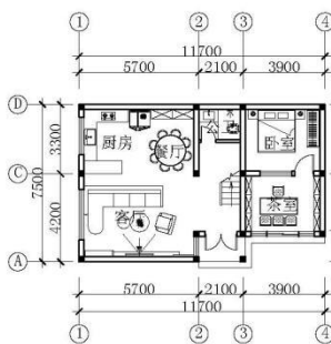
一层平面布置图 1:200
