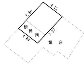
一幢三层平面图
