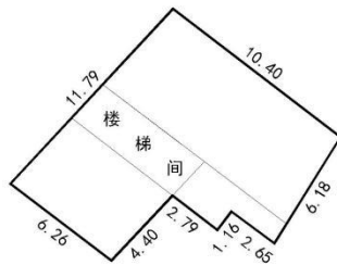
一幢一层平面图
