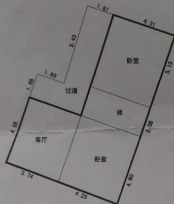
一幢一层平面图
