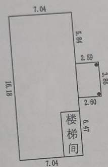
一幢一层平面图
