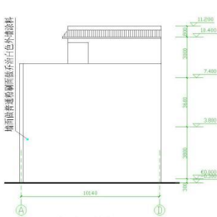
右侧立面图 1:100
