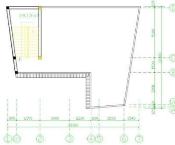
三层平面图 1:100
