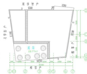
屋顶投影总平面图 1:100
