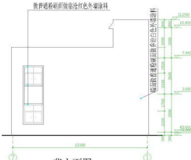
背立面图 1:100
