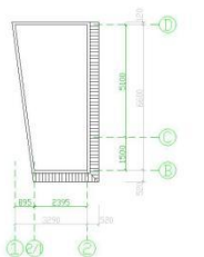
屋顶平面图 1:100
