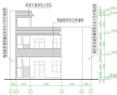
正立面图 1:100
