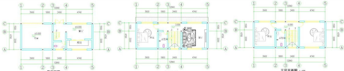
一层平面图 1:100 1. 本层面积: 104.0 平方米 2. 总建筑面积: 207.30 平方米
