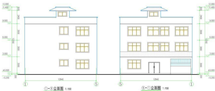
①-③立面图 1:150
