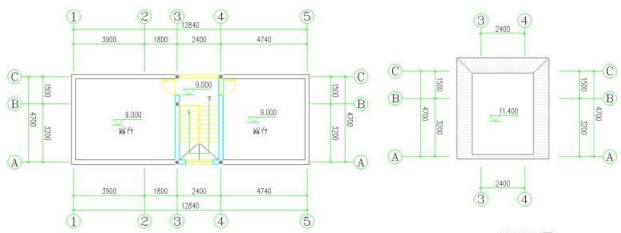
四层平面图 1:100 1. 本层面积: 104.0 平方米
