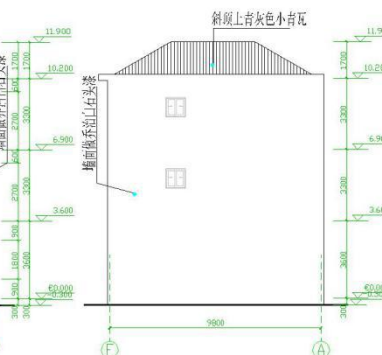
左侧立面图 1:100
