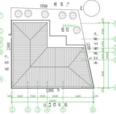
屋顶平面图 1:100
