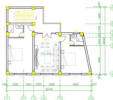
三层平面图 1:100
