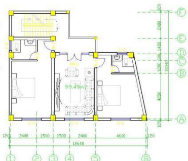
二层平面图 1:100
