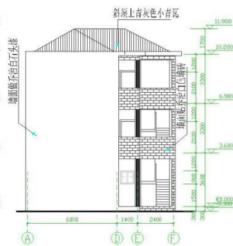
右侧立面图 1:100
