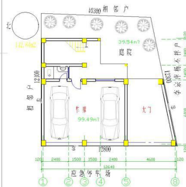
一层平面图 1:100
