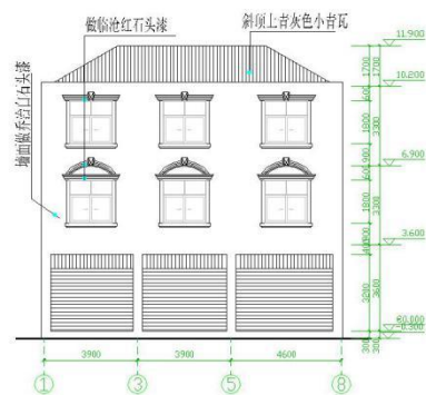
正立面图 1:100
