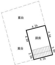
1幢4层平面图
