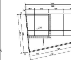
三层加盖平面图 1:100 三层加盖后建筑面积: 106.21平方米
