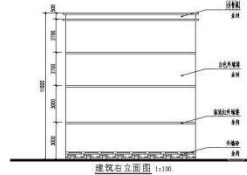
建筑右立面图 1:100
