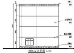
建筑左立面图 1:100
