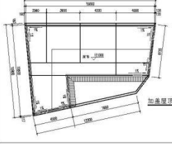
四层加盖平面图 1:100 四层加盖建筑面积: 106.21平方米
