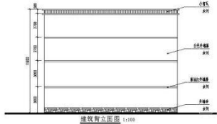
建筑背立面图 1:100
